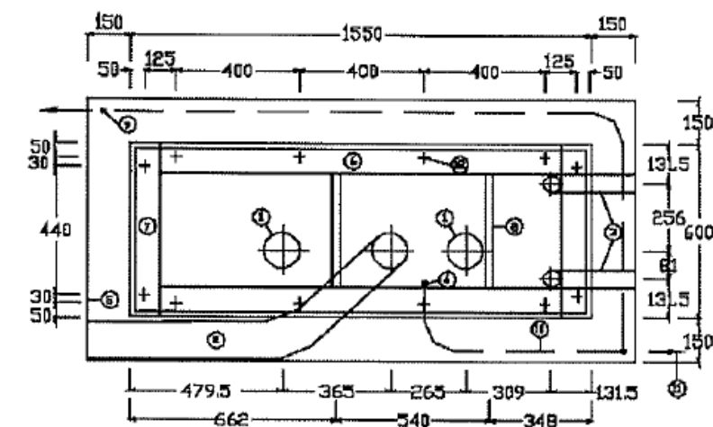
Figura 5: Esquema basament armari Tipus 2
