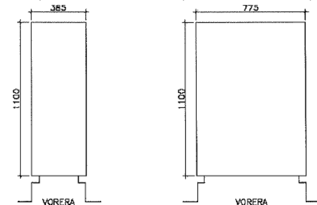
Figura 1 : Armari d'intempèrie TIPUS 1
