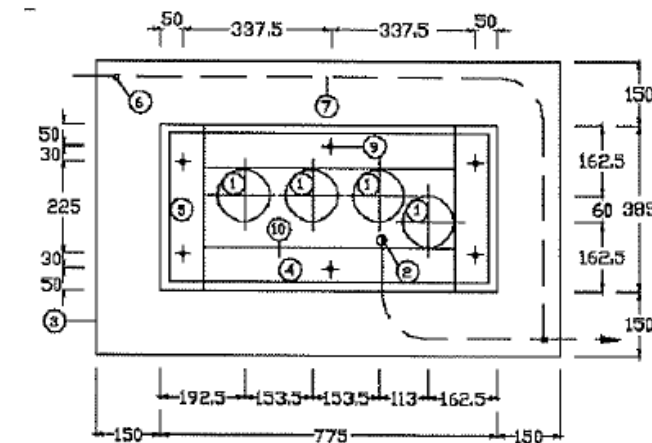
Figura 4: Esquema basament armari Tipus 1
